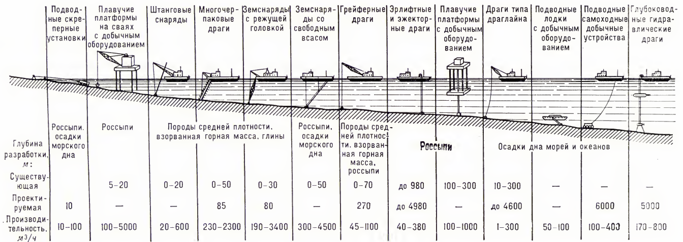
Рис. 1. Технические средства подводной добычи полезных ископаемых.
